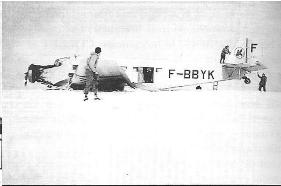
Accident du F-BBYK. Altimètre de bord 1800 m. Mont Ventoux 1909 m.
